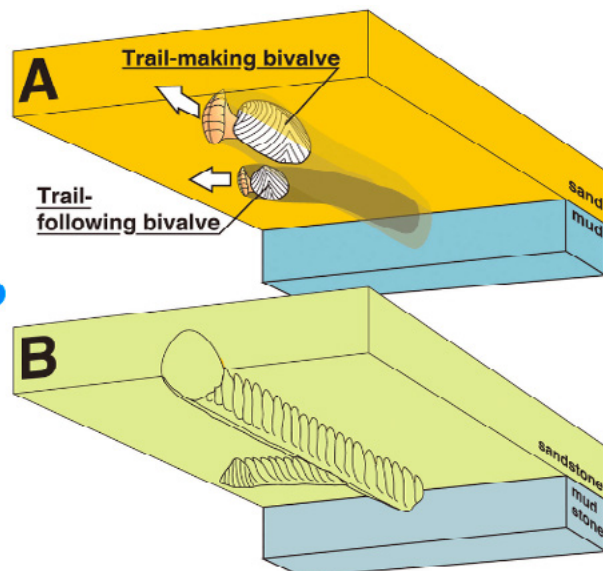
Inoceramus - foto F.Šulgan, kresba Česká geologická služba
